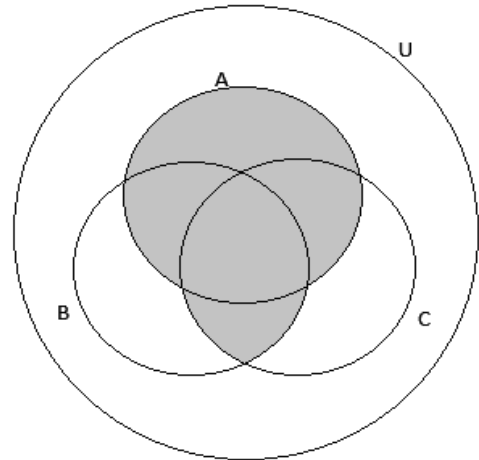
Diagrama de Euler
